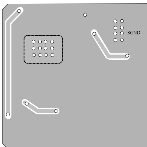
Bottom Layer
