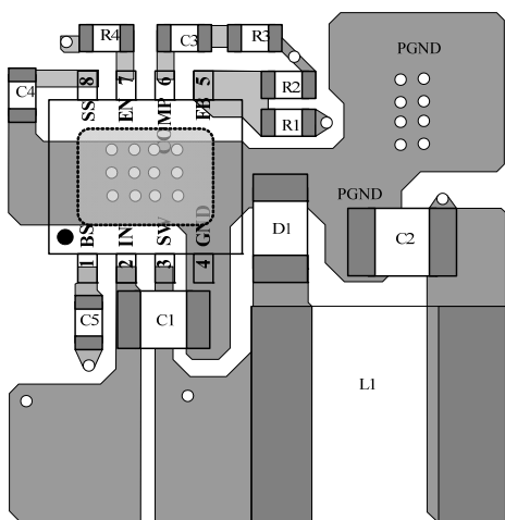
Top Layer
